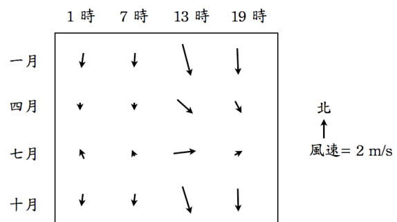
某測站長期氣候平均的近地面風向風速隨不同月份與地方時的變化 (箭號方向為風向，箭號長度與風速成正比)
